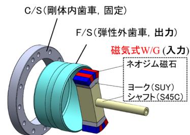
磁気式波動歯車の一例
