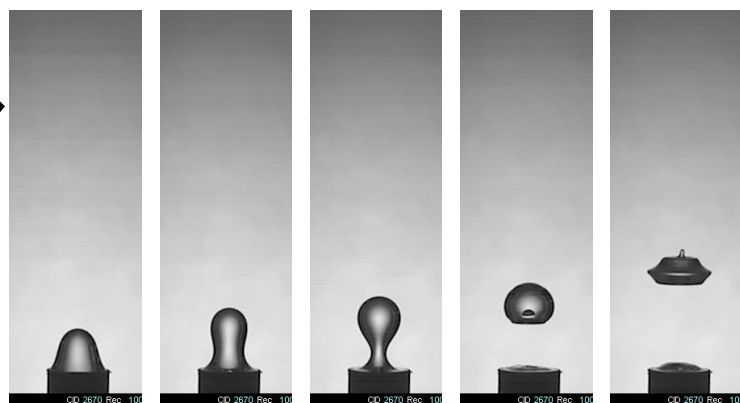
撥水面から離脱する気泡の様子
